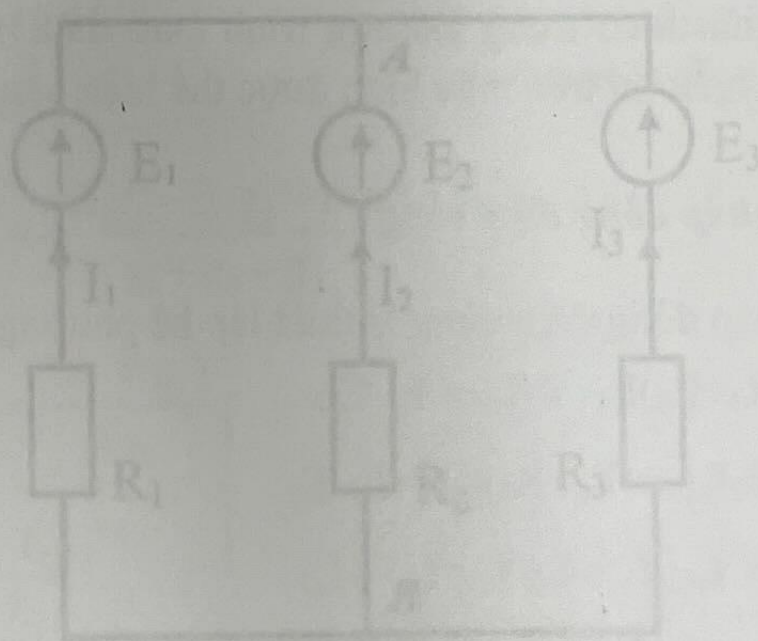
Hình 9.1a Sơ đồ mạch điện
